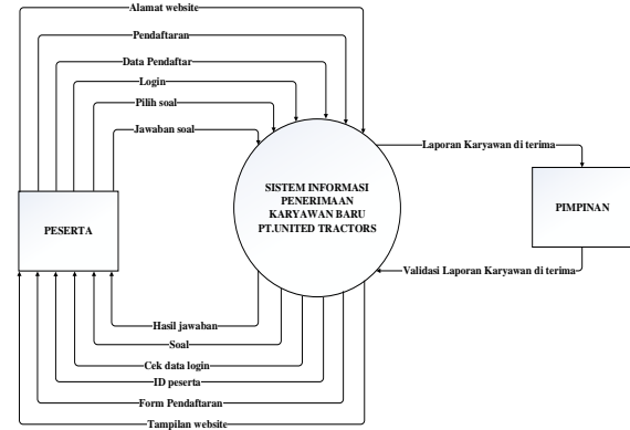
Gambar 4-3 Sistem yang di usulkan
