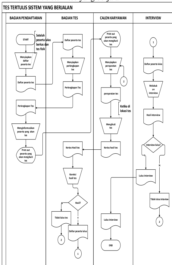
Gambar 4-2 flowchart sistem tes yang berjalan
