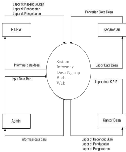
Gambar 1. Diagram Konteks
