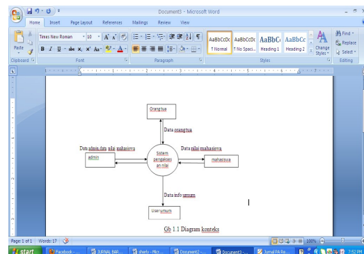
Gambar 1.1 diagram konteks
