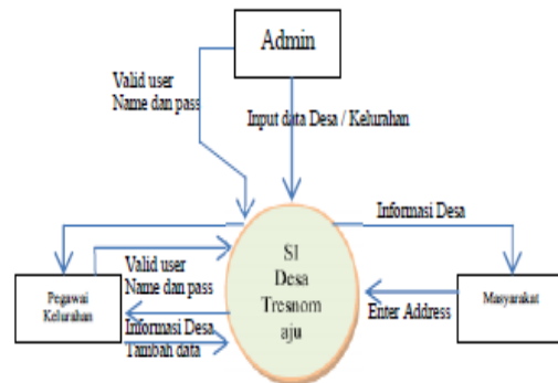
Gambar 4.2 : Bagan diagram konteks
